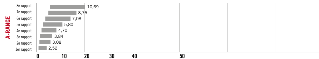
Transmission ActiveDrive 8 - Powershift 24 AV x 24 AR, 8 rapports [km/h]
